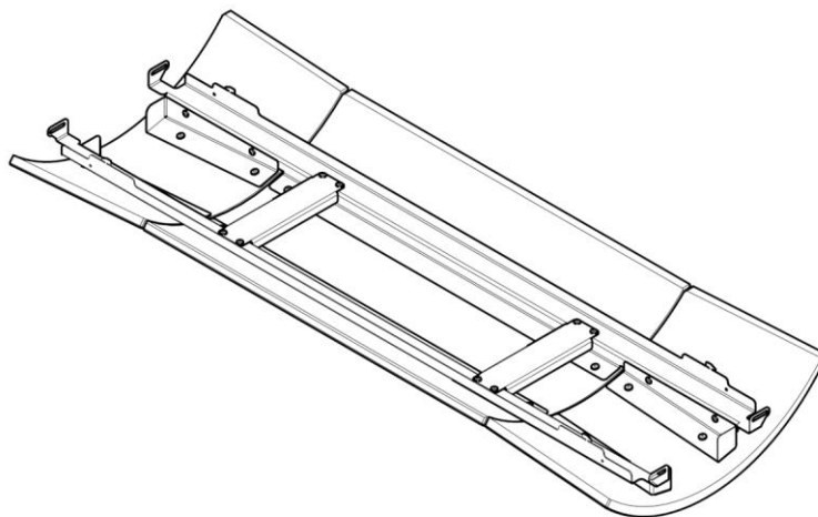
Côté assemblé
