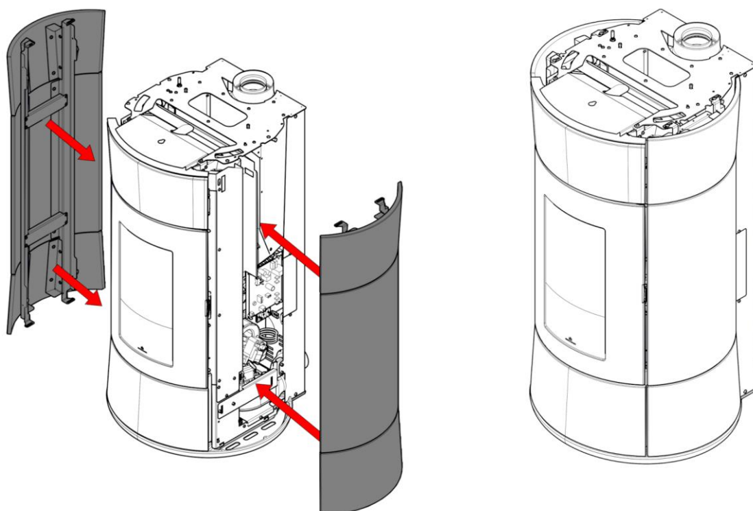
Côté assemblé
