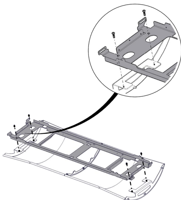
5) Positionner le support métallique
