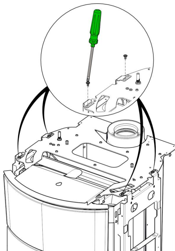
3) Dévisser les vis
