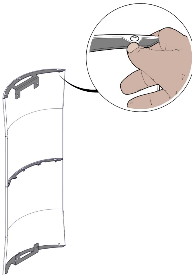
Détail positionnement étriers
