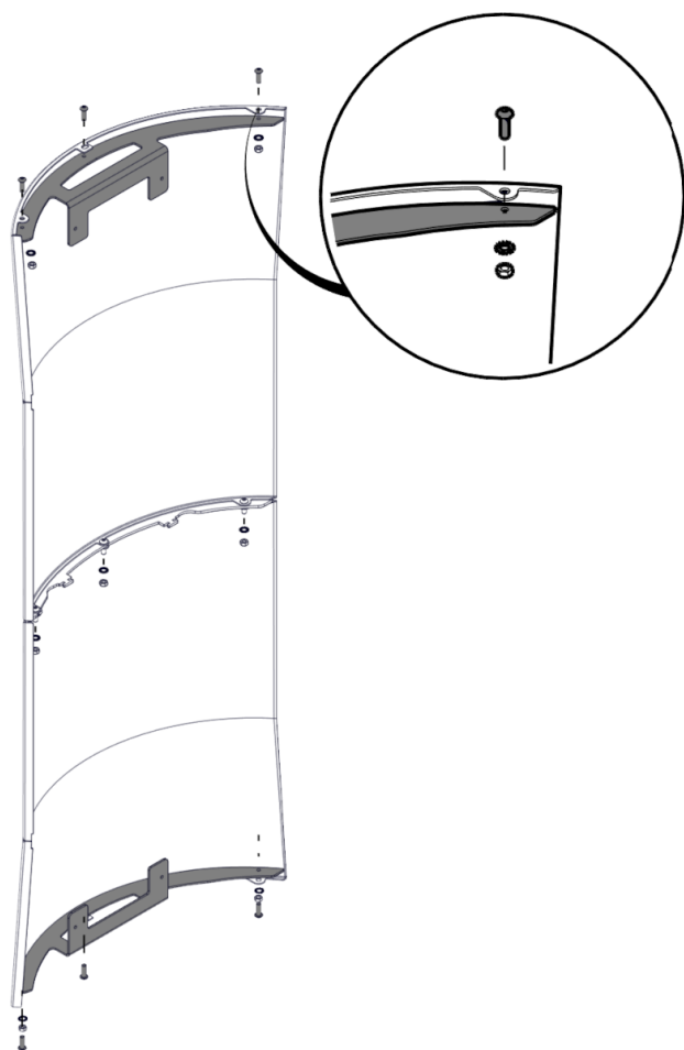
4) Positionner les étriers
