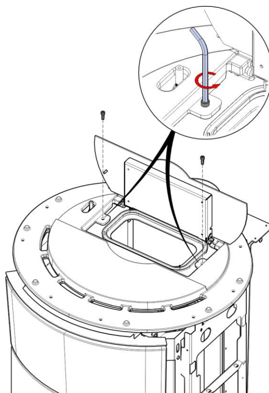
1) Ouvrir le réservoir de granulé et dévisser les vis
