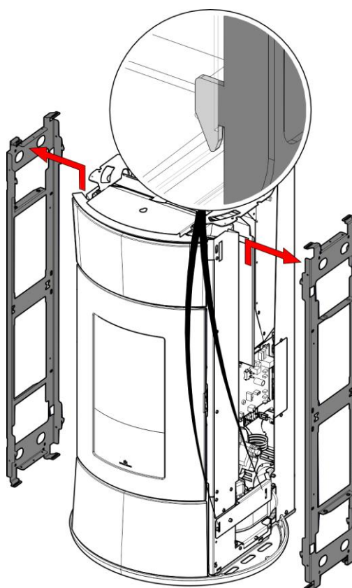
4) Côté démonté
